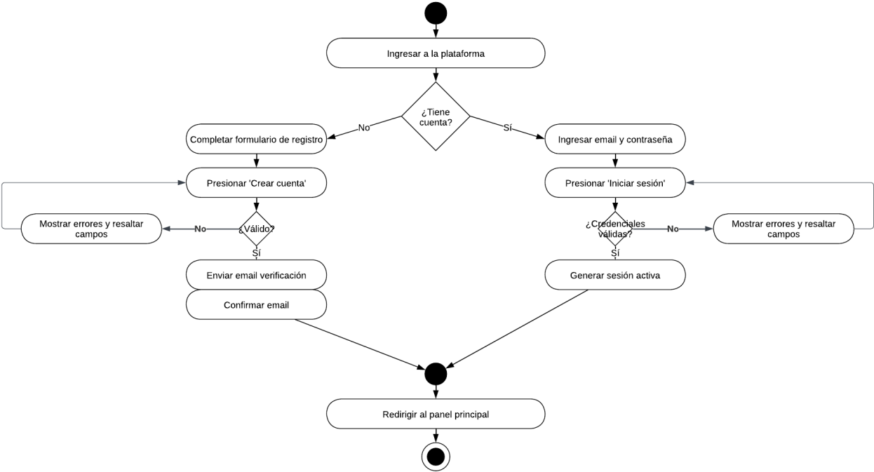
Diagrama de Actividades — RF-001: Control de acceso
