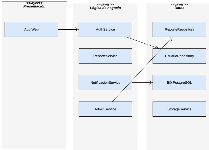
Diagrama de Componentes — Visión Barrial
