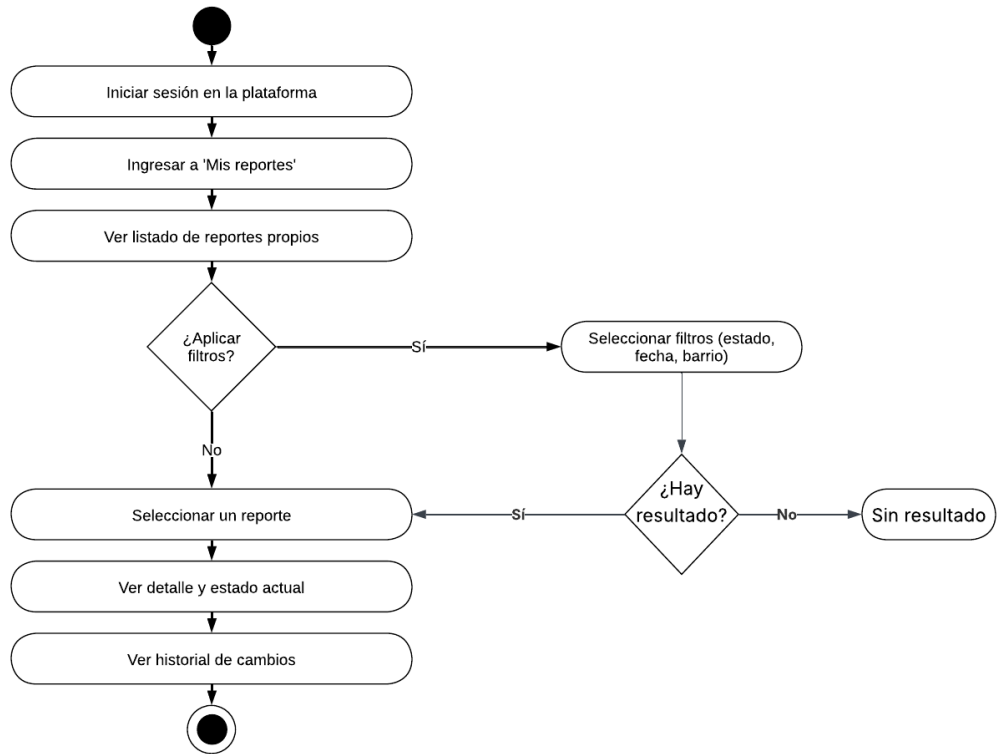
Diagrama de Actividades — RF-003: Seguimiento del reporte
