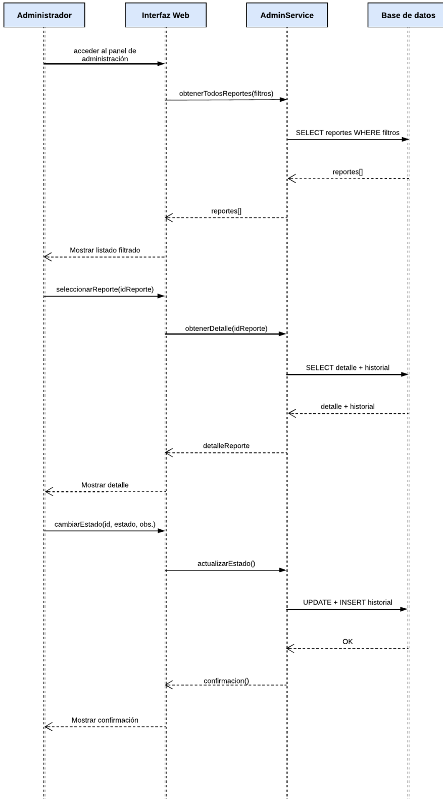
Diagrama de Secuencia — RF-004: Panel administradores
