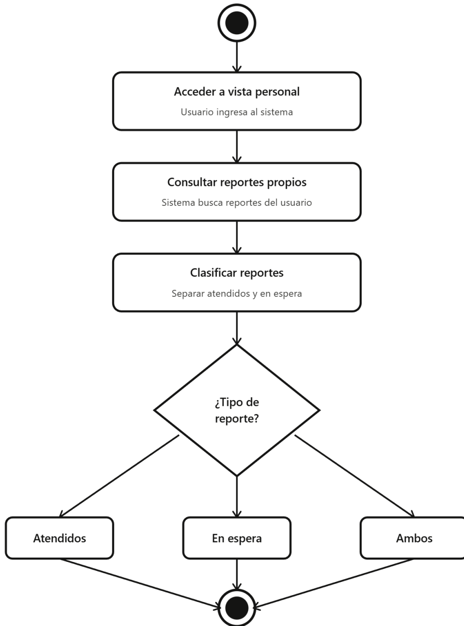
Diagrama de Actividades — RF-005: Vista del ciudadano
