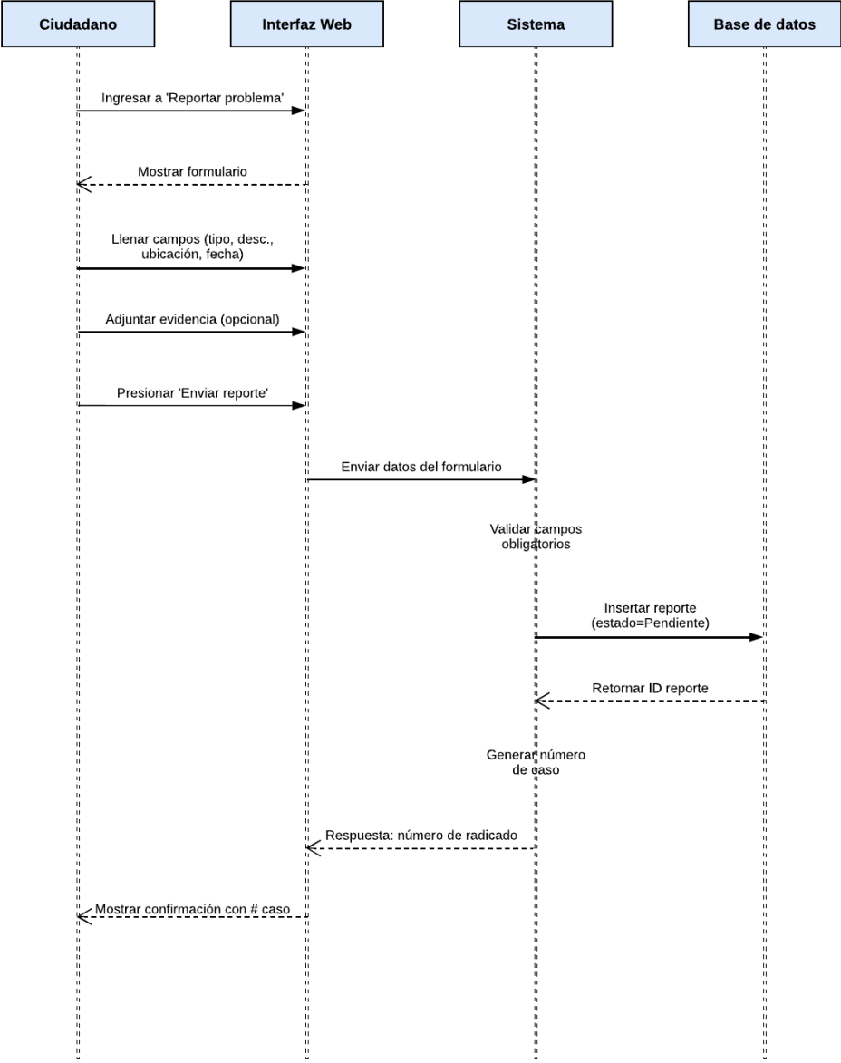
Diagrama de Secuencia — RF-002: Reportar problema
