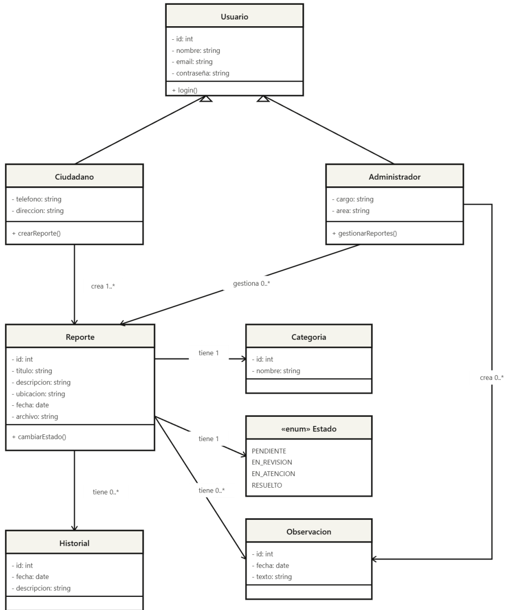
Diagrama de Clases — Sistema de Reportes Ciudadanos
