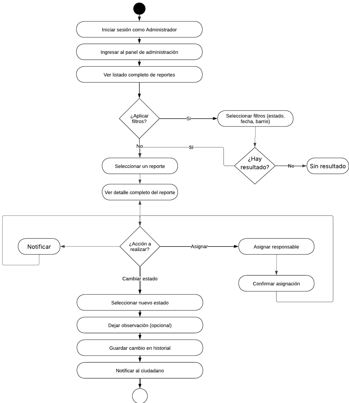
Diagrama de Actividades — RF-004: Panel administradores
